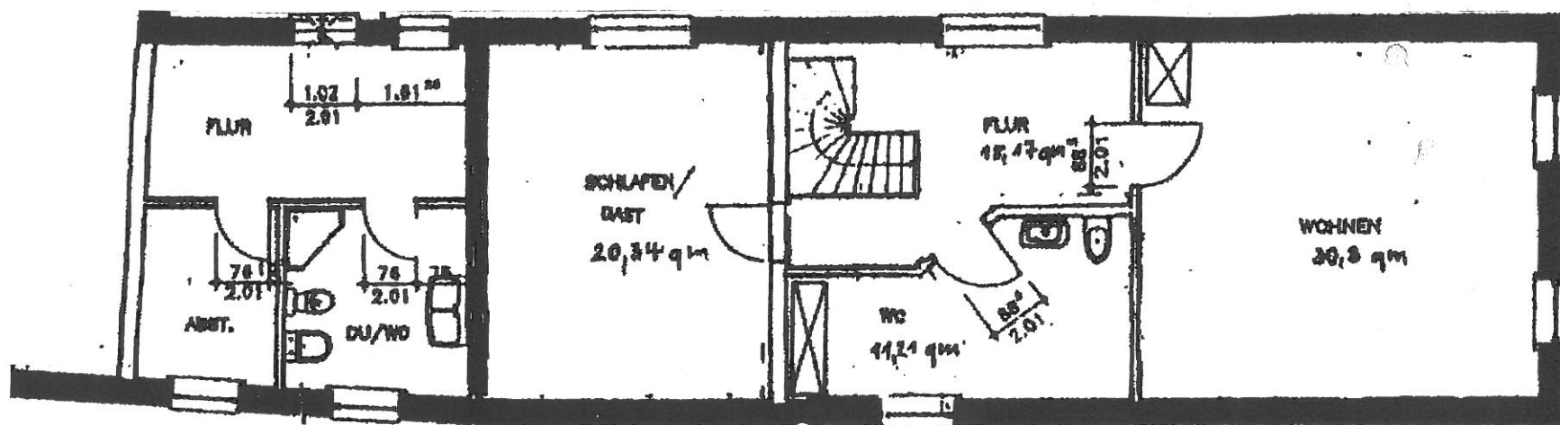
Erdgeschoss: ca. 66 m 2
